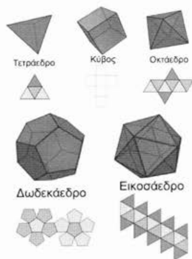
πλατωνικά στερεά
