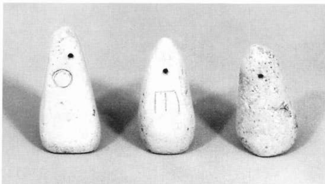
Υφαντικά βάρη
