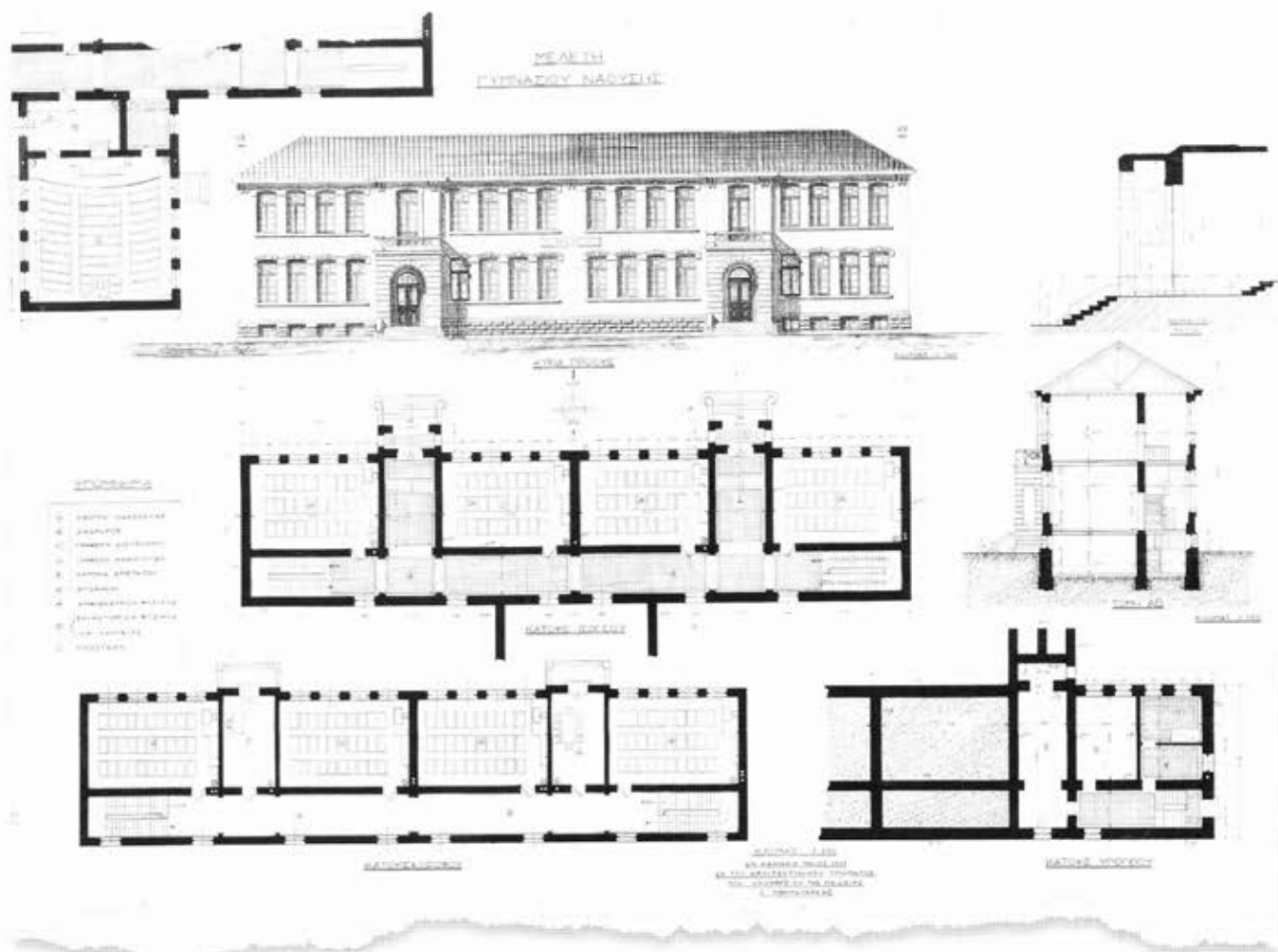
Αρχιτεκτονικό Σχέδιο του Γυμνασίου Ναούσης, το οποίο δεν κατασκευάστηκε (Αρχείο του Λαππείου Γυμνασίου)
