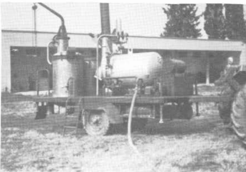
Κινητό αποστακτικό συγκρότημα
