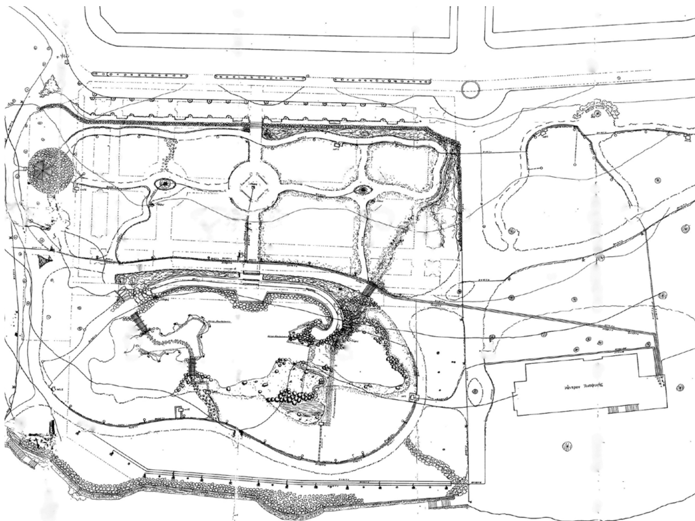
Η κάτοψη του σχεδίου του Πάρκου όπως αυτό σχεδιάστηκε από τον μηχανικό Βασίλειο Παλάσκα το 1959. Με διακεκομμένες γραμμές απεικονίζεται η αρχική κατάσταση του παρκου στην περιοχή του συντριβανιού όπως φαίνεται και στη σχετική φωτογραφία. (αρχείο Νικ. Μπάμπου)
