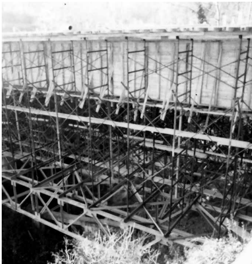
Τα μεταλλικά ικρίωματα με τα χαλύβδινα ζευκτά της νέας γέφυρας της Αράπιτσας στους Στουμπάνους
