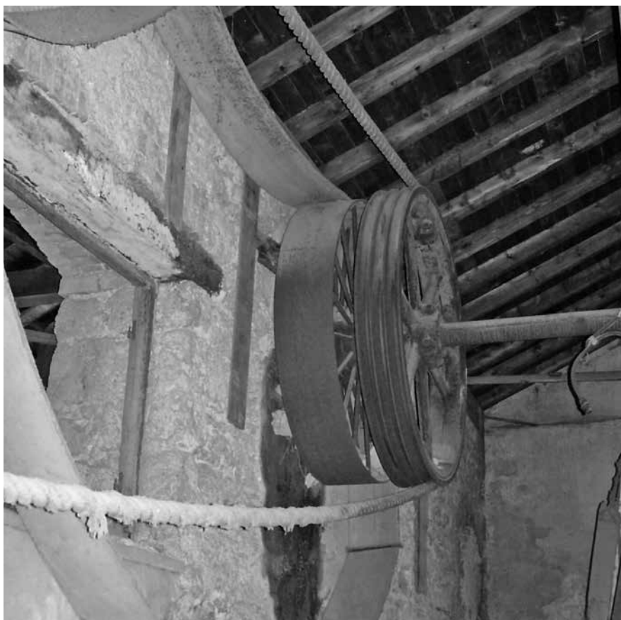
Ο κεντρικός άξονας μετάδοσης της κίνησης στα μηχανήματα του εργοστασίου μέσω τροχαλιών και ιμάντων
