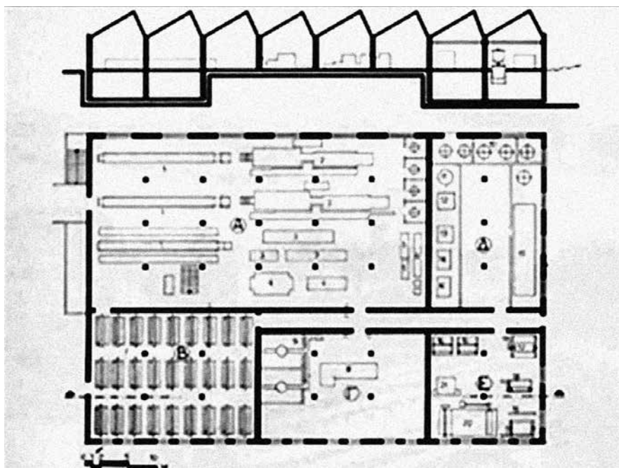
Εριουργείο ΣΕΦΕ.ΚΟ Α.Ε. Κάτοψη - τομή του κτιρίου παραγωγής. Α. Κλωστήριο, Β. Υφαντήριο, Γ. Αναμικτήριο, Δ. Βαφείο, Ε. Ξηρό φινιριστήριο (αρχείο εργοστασίου)
