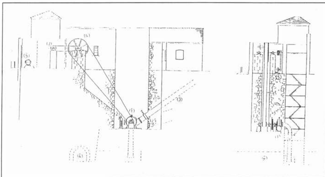
Σχεδιαστική αναπαράσταση της κεντρικής τουρμπίνας του εργοστασίου Λόγγου, Κύρση και Τουρπάλη
