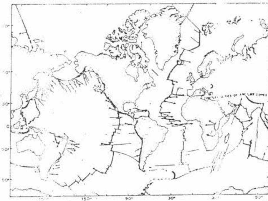
Διευθύνσεις των σχετικών οριζόντιων κινήσεων όπως προέκυψαν από την μελέτη του μηχανισμού γένεσης των σεισμών
