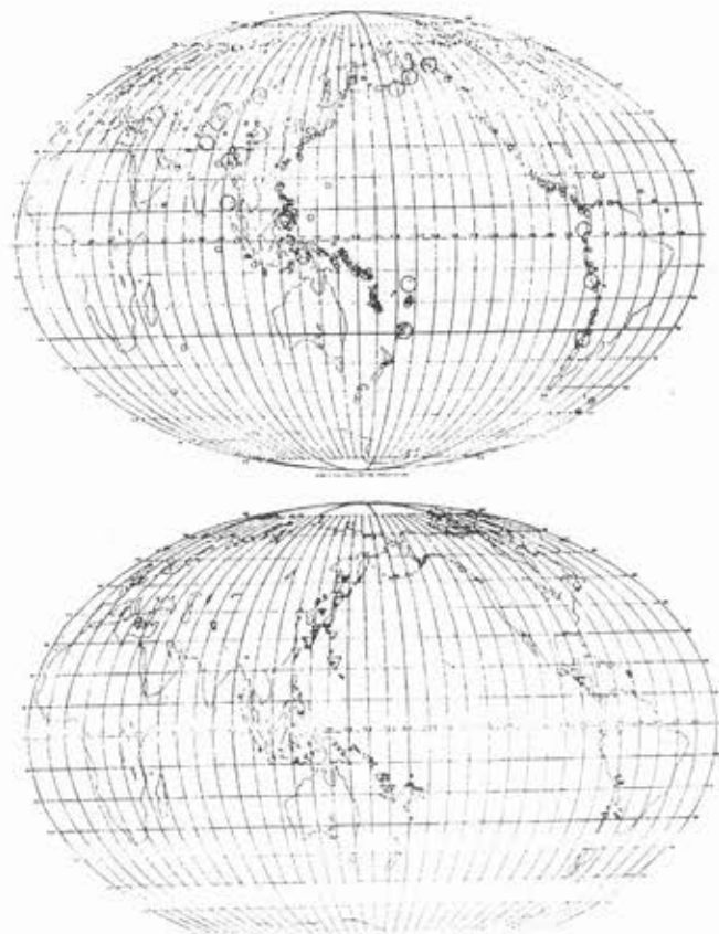
Γεωγραφική κατανομή των μεγάλων επιφανειακών σεισμών (πάνω) και των πλουτώνιων σεισμών (κάτω), (Richter 1958)
